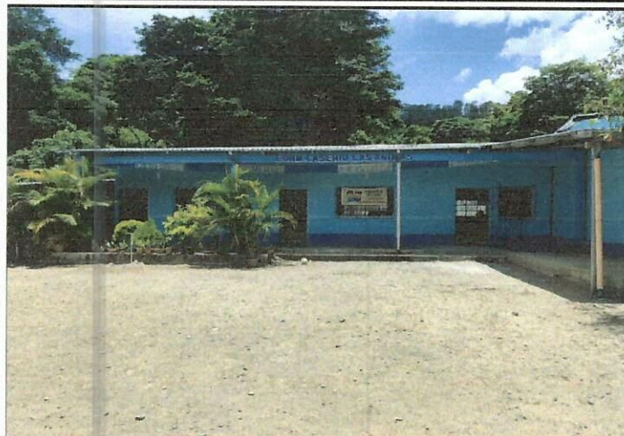
Foto 1: Mejoramiento de Estructura de techo con Tubo Galvanizado Chapa 14, con cubierta de lámina calibre 26.
